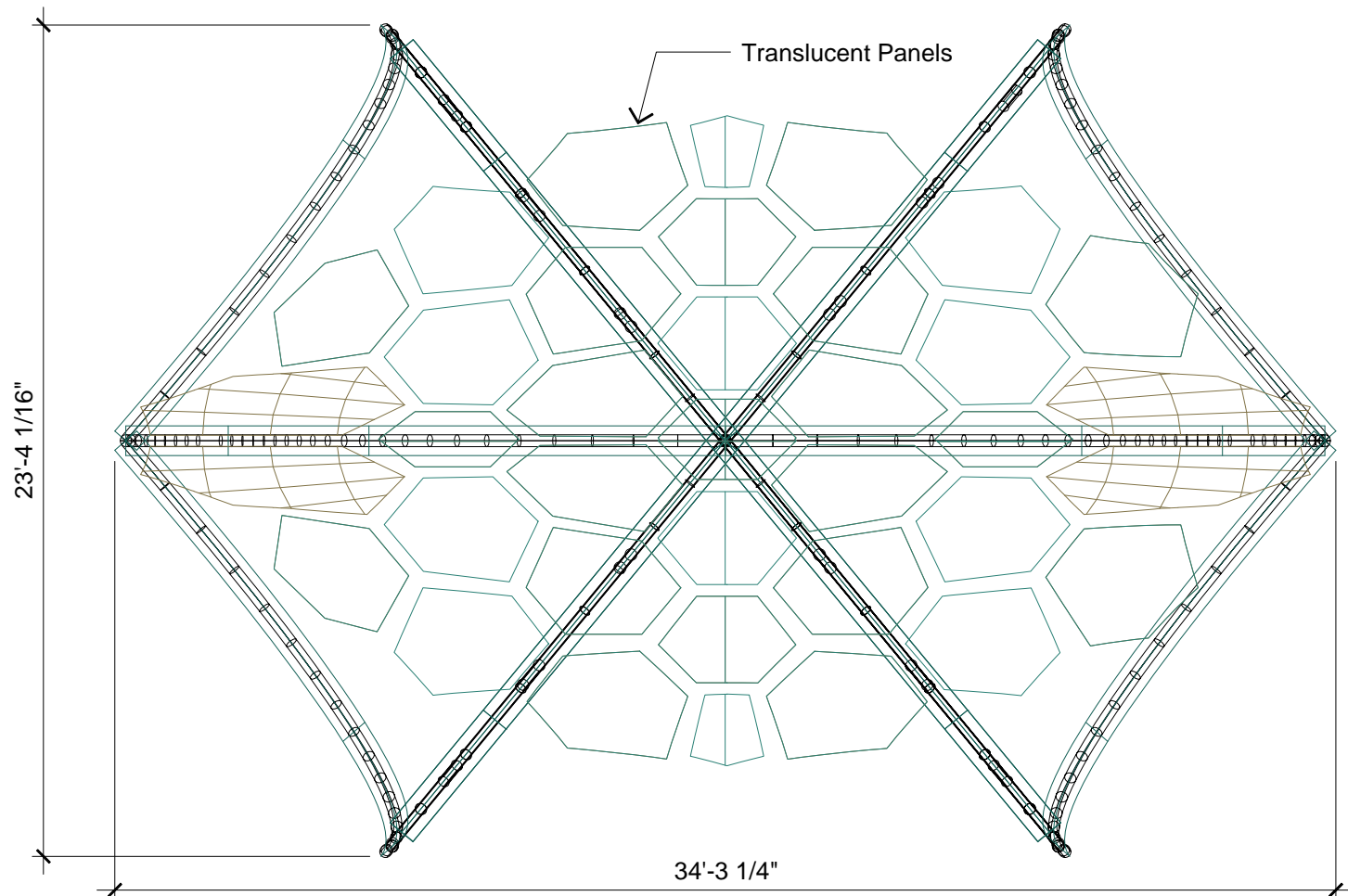
2 TURTEL POD TOP SCALE: 1:60
